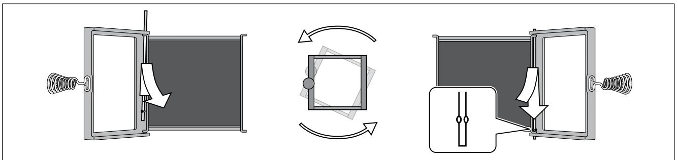
Рисунок 11. Изменение стороны подвески дверцы каменки
