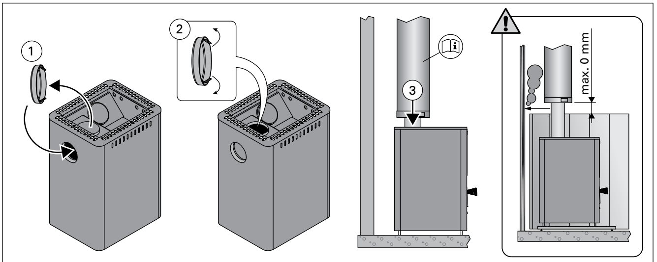
Рисунок 10. Присоединение печи к стальному дымоходу Harvia (все размеры приведены в миллиметрах)
